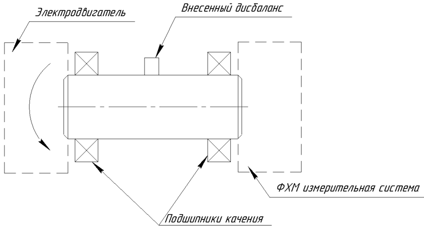
Рис. 2. Модель вращающегося вала с эксцентриситетом
