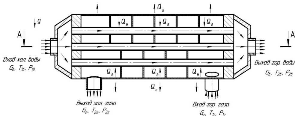
Рис. 2. Расчетная схема рекуперативного ТА
