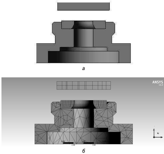
Рис. 8. 3D-модель клапана и Сетка конечных элементов для моделирования
