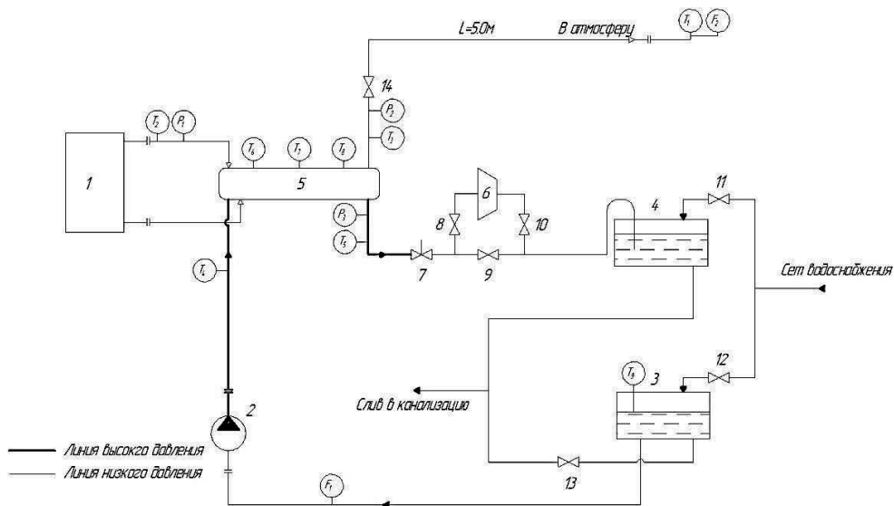
Рис. 4. Схема функциональная экспериментального стенда для исследования ТА: 1 — ДВС; 2 — плунжерный насос; 3, 4 — бак; 5 — теплообменник; 6 — объемный расширительный агрегат; 7 — регулирующий вентиль; 8, 9, 10, 11, 12, 13, 14 — краны
