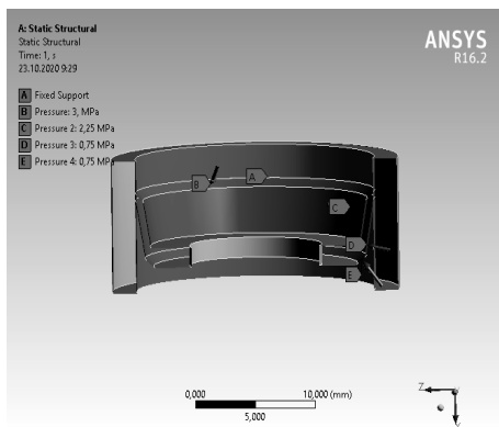
Рис. 11. Граничные условия
