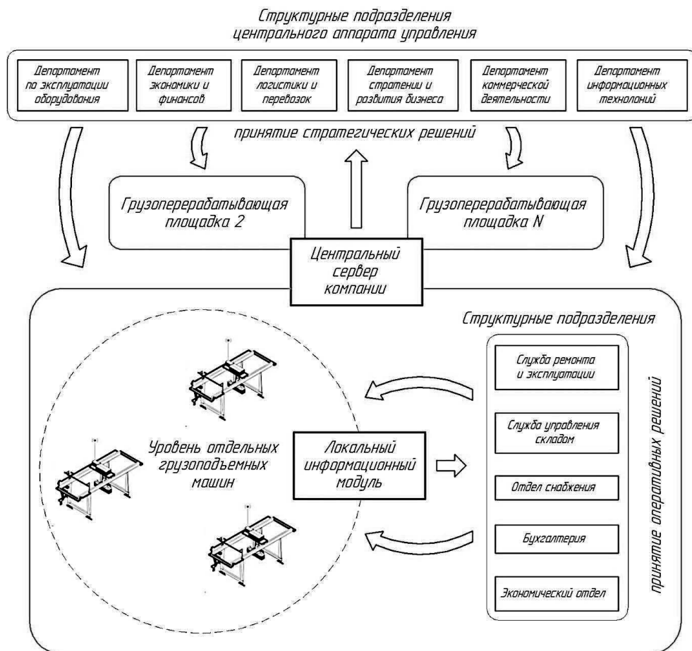
Рис. 4. Схема иерархической информационно-управляющей системы
