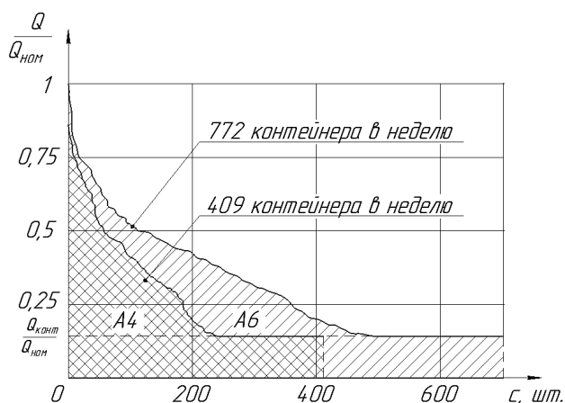
Рис. 3. Результаты расчета интенсивности эксплуатации оборудования на контейнерном терминале при определенных колебаниях интенсивности грузопотока ( Q_{\text{конт}} — масса пустого контейнера)
