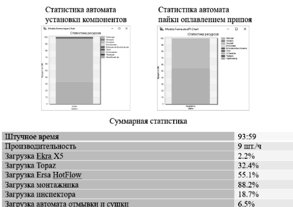
Рис. 3. Пример результатов работы модуля Plant Simulation
