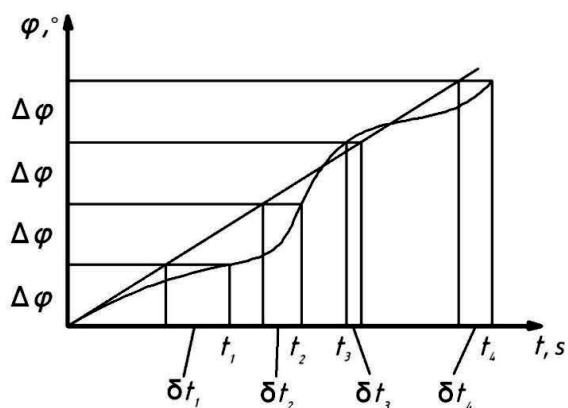
Рис. 1. Принцип работы фазохронометрической системы
