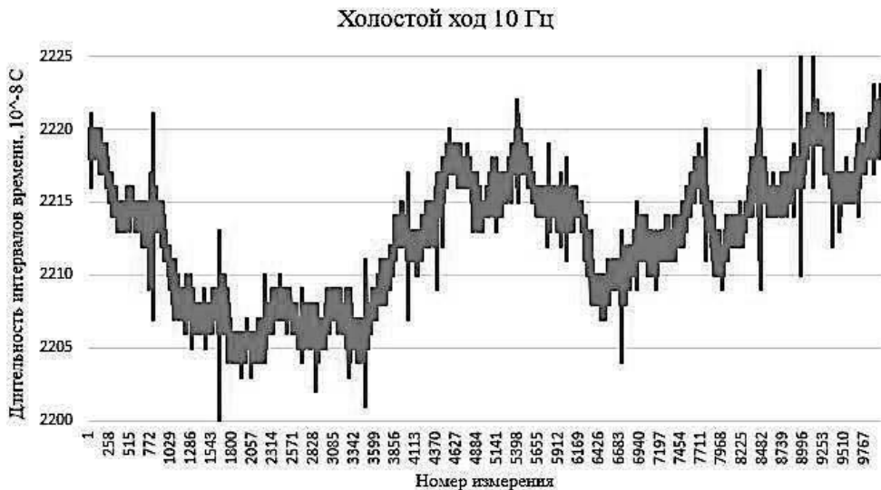
Рис. 3. Хронограмма вращения квазиуравновешенной системы
