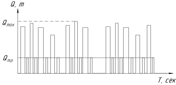
Рис. 1. Экспериментальная циклограмма работы контейнерного крана:
