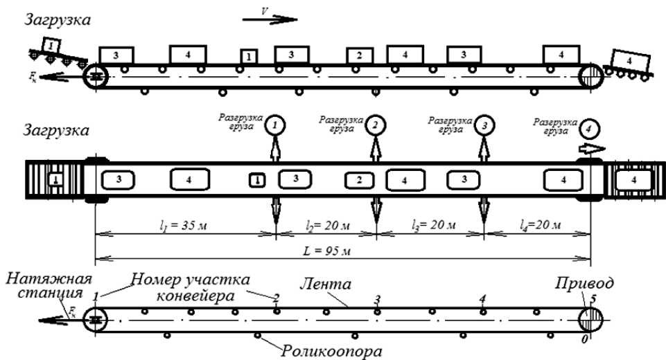
Рис. 1. Схема ленточного конвейера
