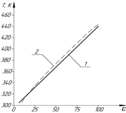
Рис. 6. График изменения средней температуры нагнетаемого газа без интенсивного охлаждения ступени при t=2 с: 1 — эксперимент; 2 — цифровой двойник
