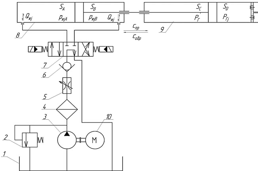
Рис. 1. Расчетная схема гидравлического привода
