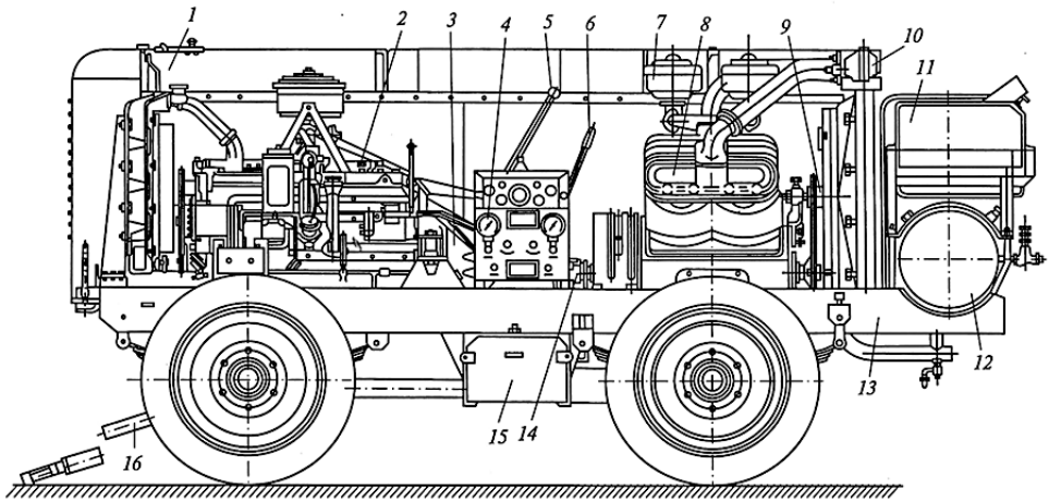
Рис. 1. Передвижная мобильная компрессорная установка ПКС-5:
