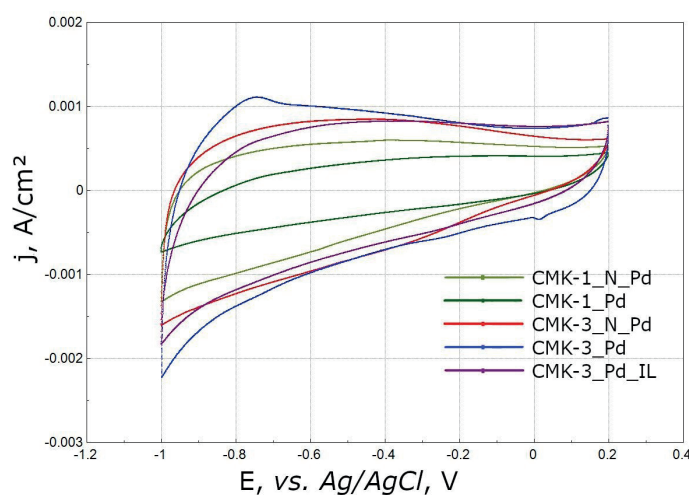
Рис. 4. Циклическая вольтамперограмма (ЦВА) на электроде с различными катализаторами в деаэрированном 0.1 М растворе \text{KOH} : скорость развертки потенциала 50 \text{ mV} \cdot \text{s}^{-1} .
