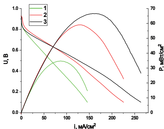
Рис. 11. Вольтамперные кривые и зависимость плотности мощности от плотности тока для МЭБ ШТЭ с катодами на основе катализатора 7% Pd/CMK-3: 1 – 0.4 мг Pd /см 2 (степень сжатия катода 20%); 2 – 0.4 мг Pd /см 2 (степень сжатия катода <10%); 3 – 0.07 мг Pd /см 2 (степень сжатия катода <10%). В качестве анодного катализатора во всех случаях использовался PtMo/УНТ (0.4 мг Pt /см 2 ). 40°C, RH=100%, ГДС 39 ВВ, I/C=1/1.
