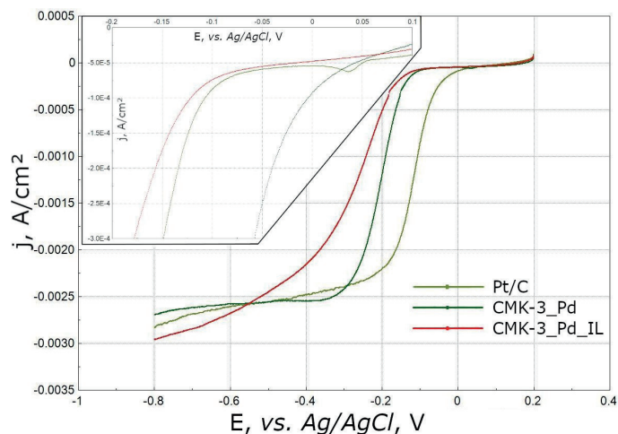
Рис. 5. Вольтамперограммы наиболее активных катализаторов на основе \text{CMK} и промышленного платинового катализатора: скорость развертки потенциала 5 \text{ mV} \cdot \text{s}^{-1} , скорость вращения электрода 1000 об/мин, загрузка катализатора 80 \text{ мкг} \cdot \text{см}^{-2} .
