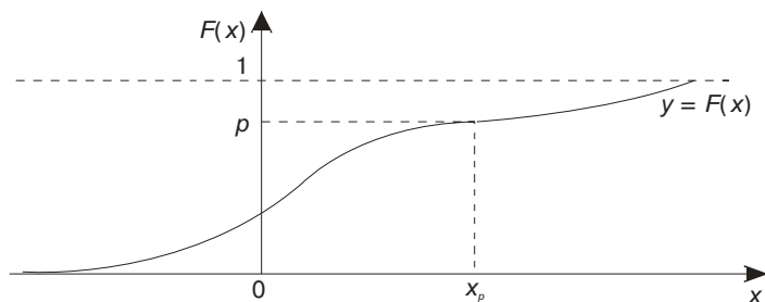
Рис. 4.2. Определение квантили x_p порядка p
