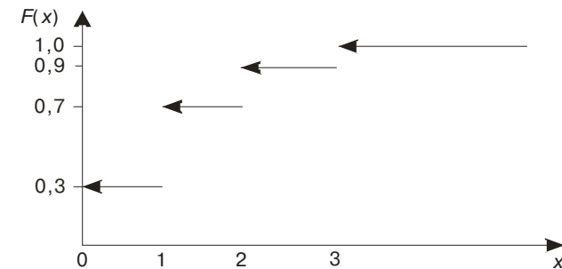
Рис. 4.1. График функции распределения числа дефектных изделий
